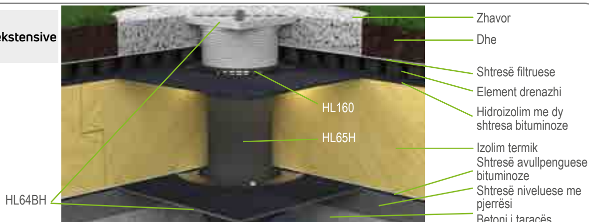
Taracë e gjelbër intensive me pusetë drenazhimi dhe inspektimi
