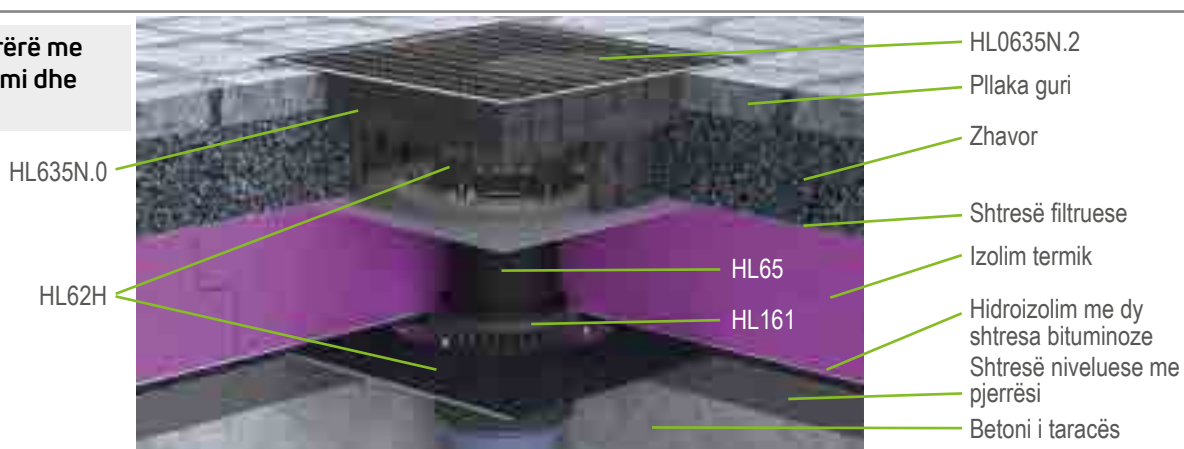
Taracë e gjelbër intensive me pusëtë drenazhimi dhe inspektimi
